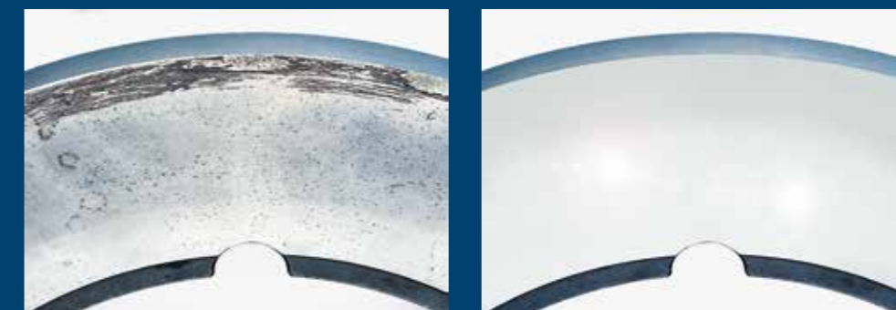
Exemple de comparaison entre deux lames de cisaille à molette : après le processus de coupe et après le polissage.
